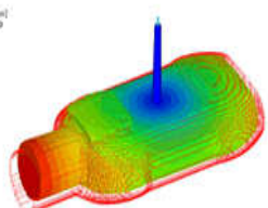
そり解析
