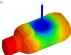
充填解析
