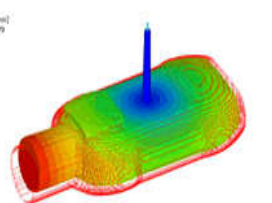
そり解析
