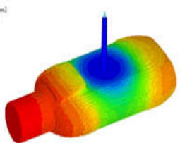
充填解析
