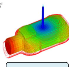
そり解析
