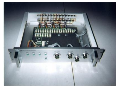
各種小型ユニットの組立配線
