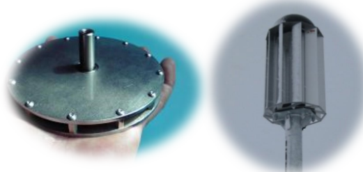
風力発電用発電機完成
